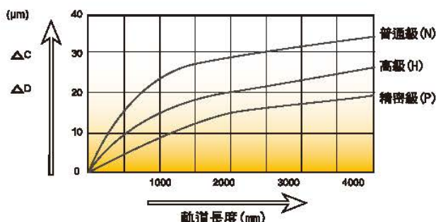
圖 1.6.1 ABBA線性滑軌的行走精度
