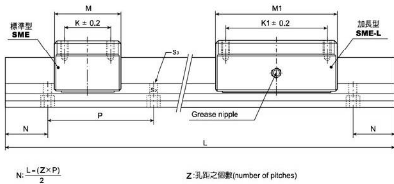
SAFB軸心式滑軌(支撐座單元)
